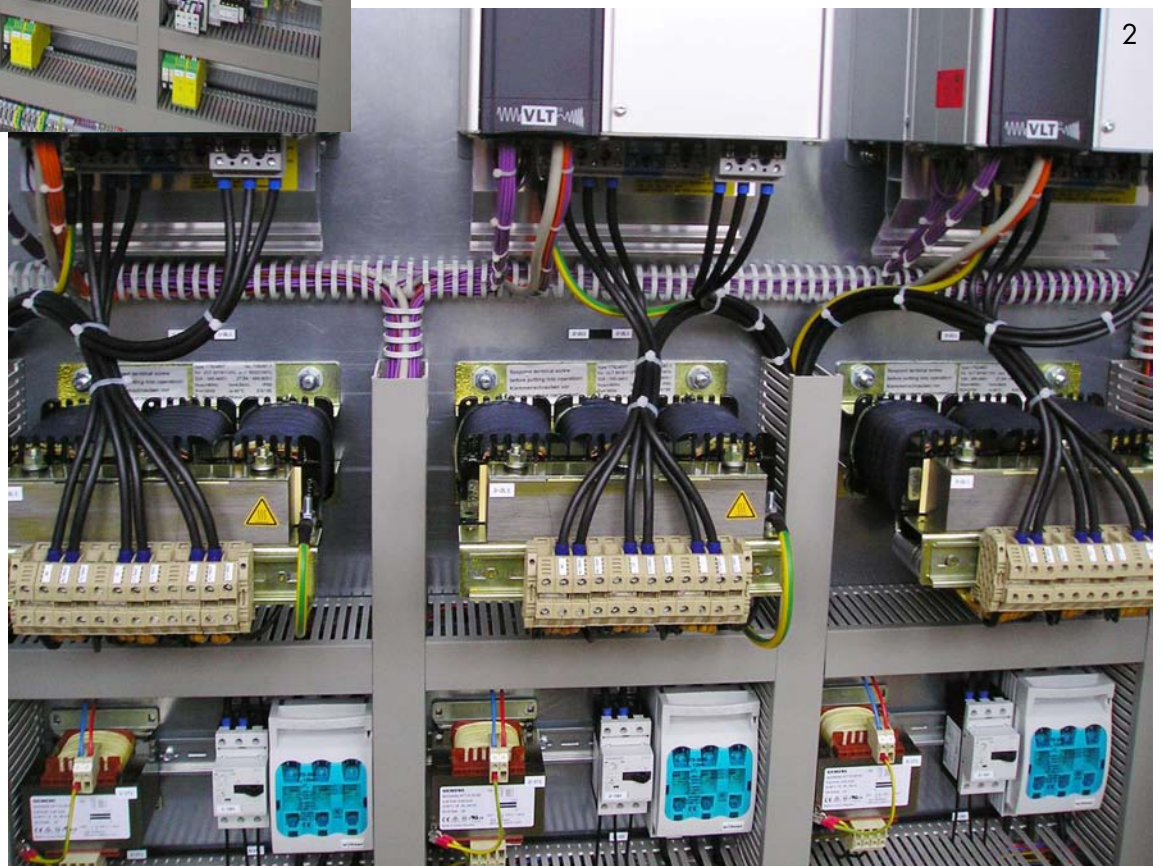
Abb. 2: Detailansicht
